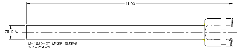
M-1580-QT MIXER SLEEVE 161-224-W
