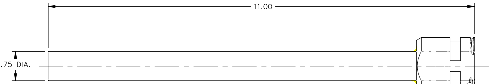
M-1580-QT MIXER SLEEVE 161-224-W
